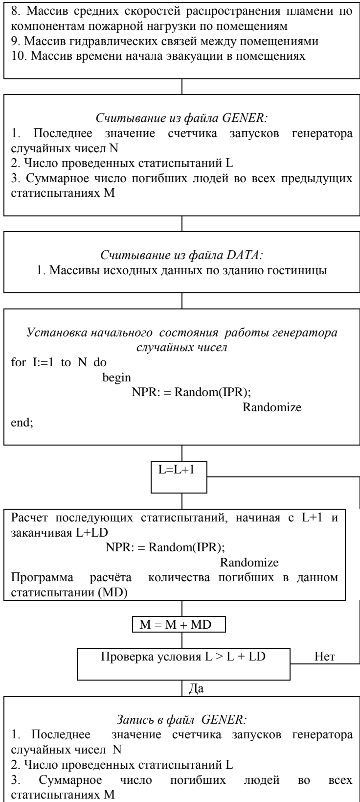
Рис 1. Структурная схема расчета Рнеэв методом статиспытаний (Монте-Карло)
